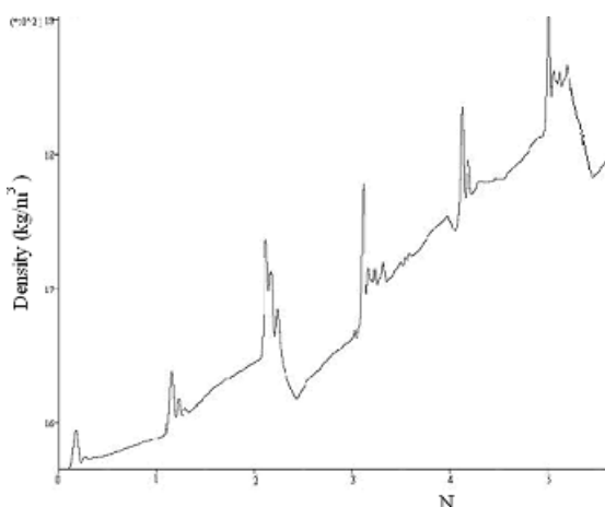
شکل (۱۹): تغییرات دانسیته در عمق بهبود در ضربات متوالی
