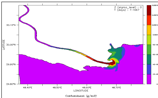
شکل ۱۰. میدان آلودگی ۱۷۴ ساعت بعد از آغاز پخش در حالت کم آبی
