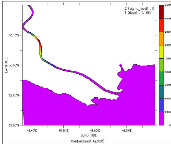
شکل ۱۳. میدان آلودگی ۳۰ ساعت بعد از آغاز پخش در حالت پراپی
