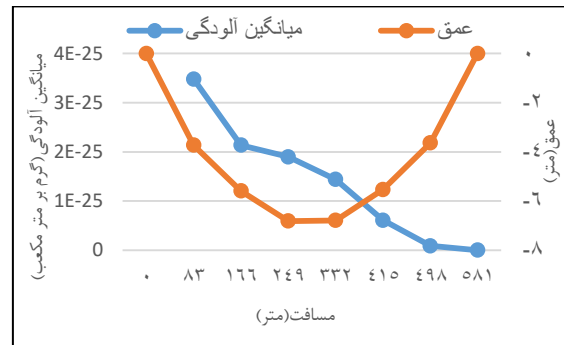
شکل ۲۱. مقطع عرضی در بالادست رودخانه برای آلودگی
