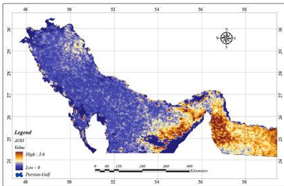
باند ۵ (۱/۲۴۳ میکرومتر)
