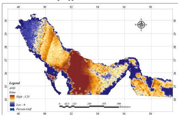
باند ۲ (۰/۸۵۵ میکرومتر)
