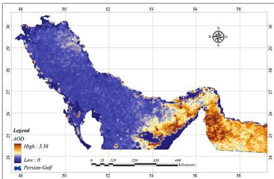
باند ۶ (۱/۶۴۳ میکرومتر)
