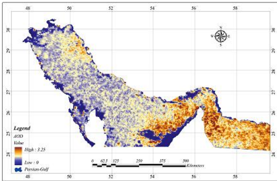
باند ۲ (۰/۸۵۵ میکرومتر)
