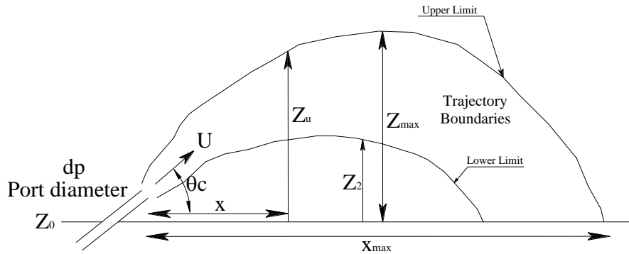
شکل ۲. نمایش پارامترهای موثر بر حرکت جریان جت
